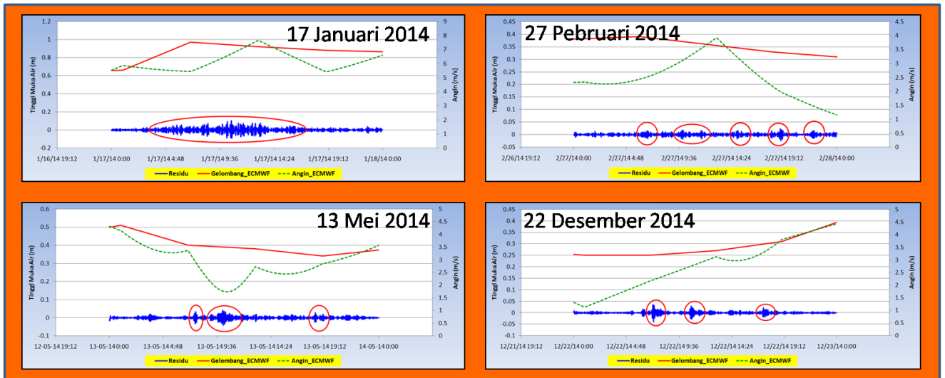
Gambar 12 Hasil Pengolahan Data Pada Tanggal Terjadinya Banjir Rob Tahun 2014
