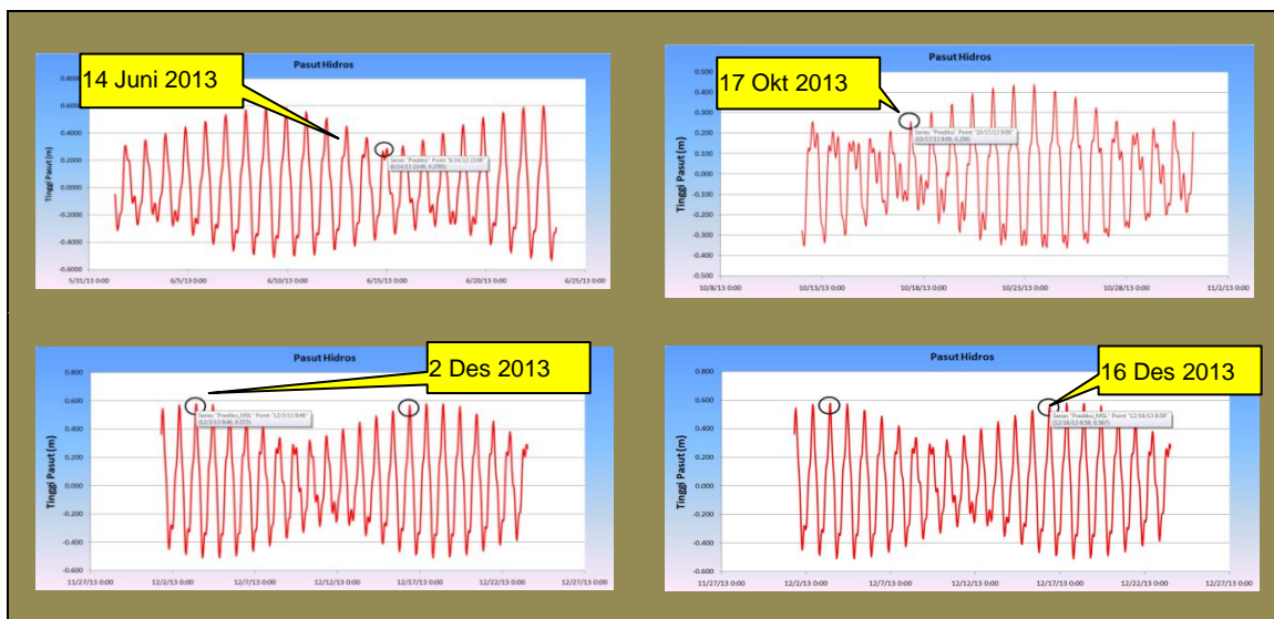
Gambar 8 Elevasi Muka Air Pasang Surut Pada Bulan Terjadinya Banjir Rob Tahun 2013
