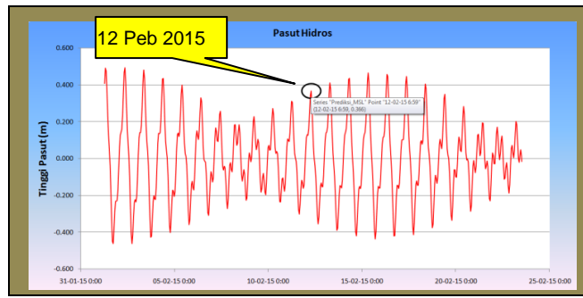
Gambar 10 Elevasi Muka Air Pasang Surut Pada Bulan Terjadinya Banjir Rob Tahun 2015
