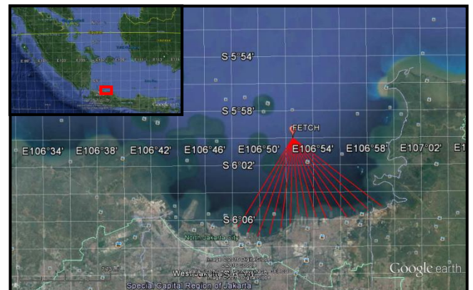
Gambar 3 Penghitungan Panjang Fetch
