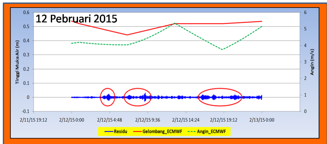
Gambar 13 Hasil Pengolahan Data Pada Tanggal Terjadinya Banjir Rob Tahun 2015
