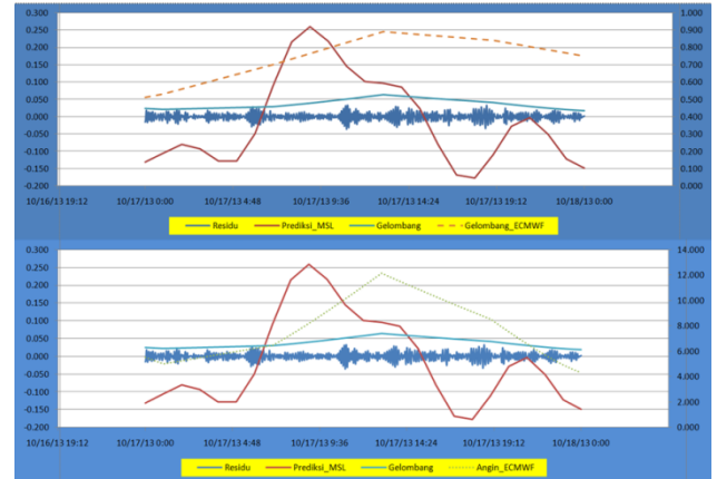
Gambar 6 Contoh Grafik Pengolahan DataKomponen Penyebab Banjir Rob
